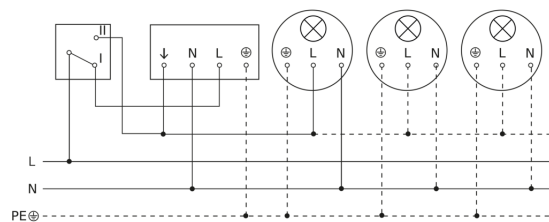
Diagrama electrónico conexión del acoplador pulsador de 4 vías al APC DALI2
