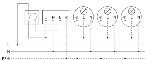
Diagrama electrónico conexión mediante interruptor en serie para funcionamiento manual y automático
