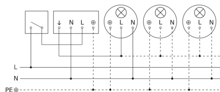
Diagrama electrónico lámpara con conductor neutro
