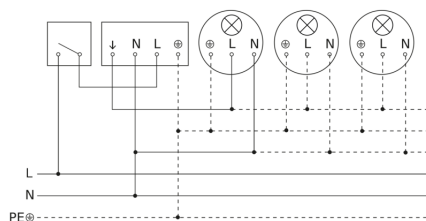
Diagrama electrónico lámpara sin conductor neutro
